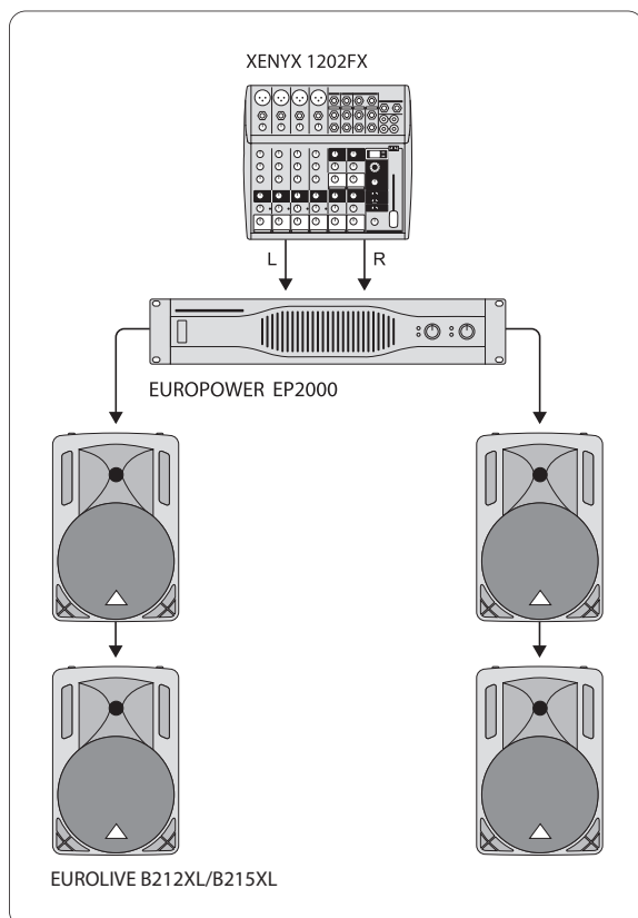
Bild 5.2: Kabeldragning för flera B212XL/B215XL
