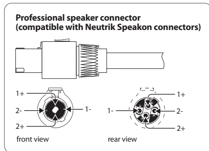
Bild 6.1: Högtalaranslutningar
