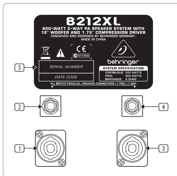
Bild 2.1: Anslutningar (B212XL och B215XL)
