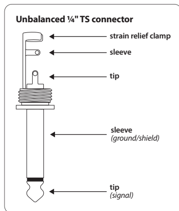
Bild 6.2: 6,3-mm-mono-jackkontakt
