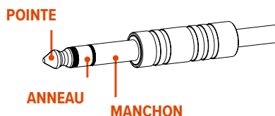
CONNECTEUR JACK TRS Câblage mono symétrique
