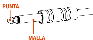
CONECTOR TRS Cableado mono no balanceado
